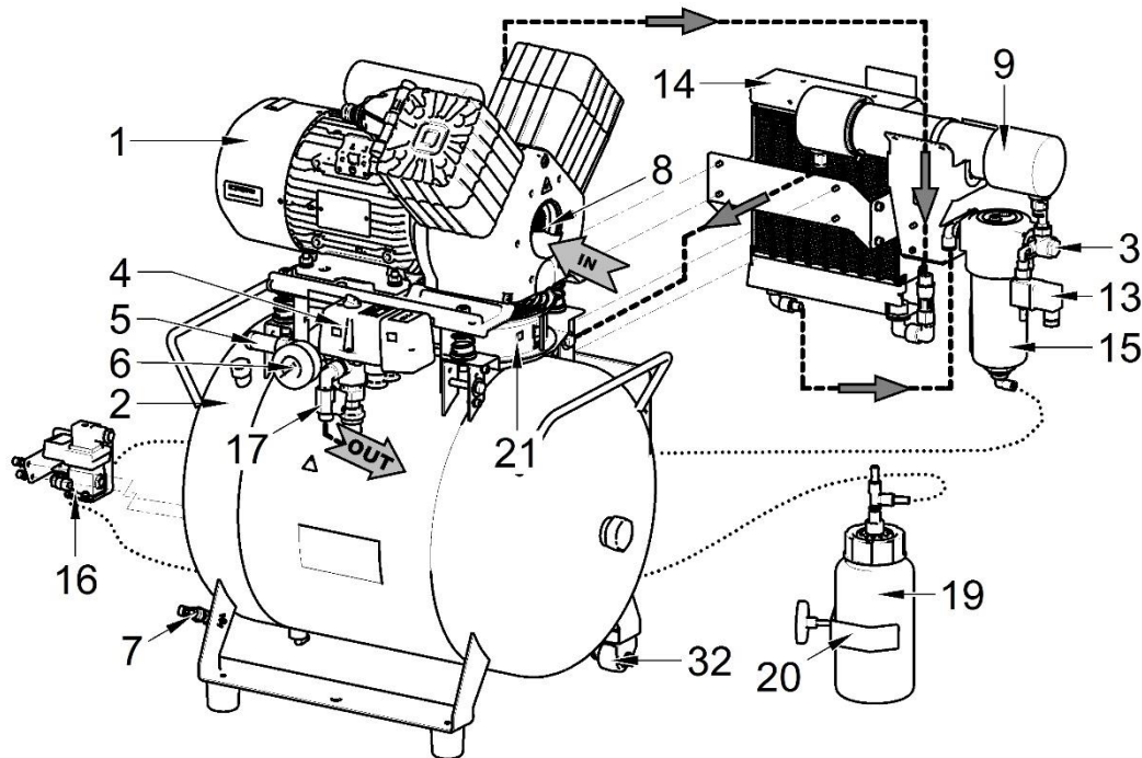
Abb. 1 - Kompressor mit Trockner
