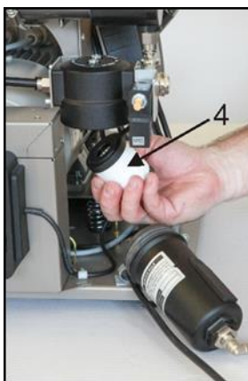
Obr. 9: Výmena filtračnej vložky vo filtri
