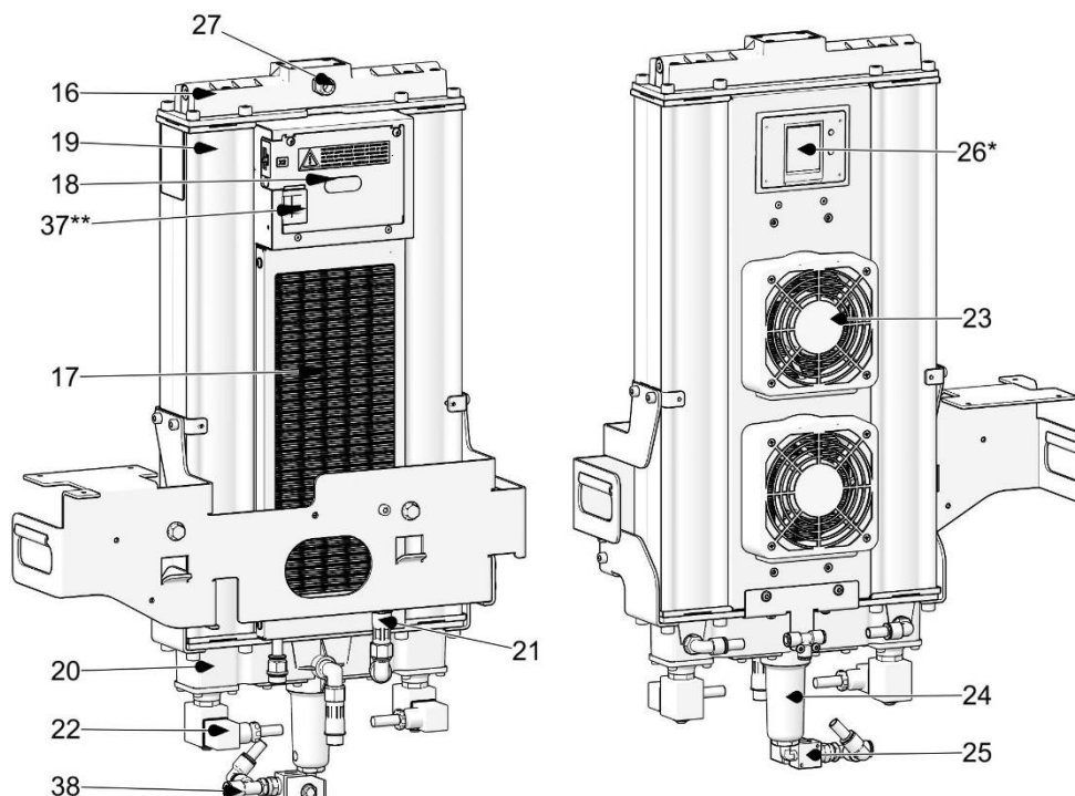
Obr. 3: Adsorpčný sušič
