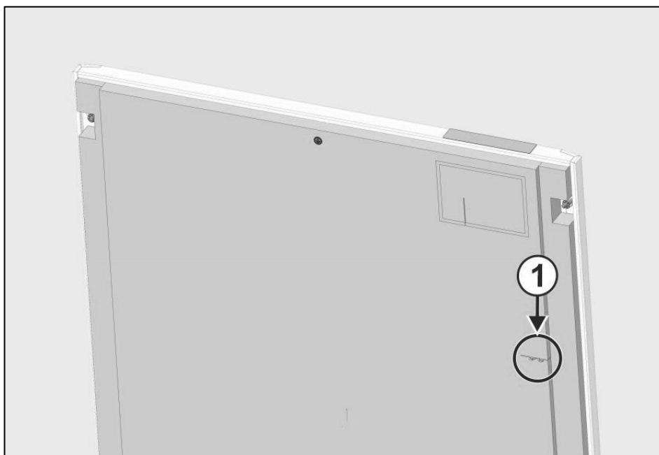
Obr. 18: Príchytky skrinky DK50 4VR/50 S/M
