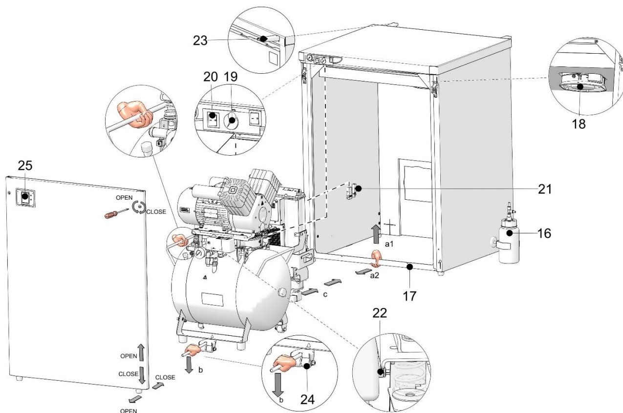
Abb. 4: Gehäuse
