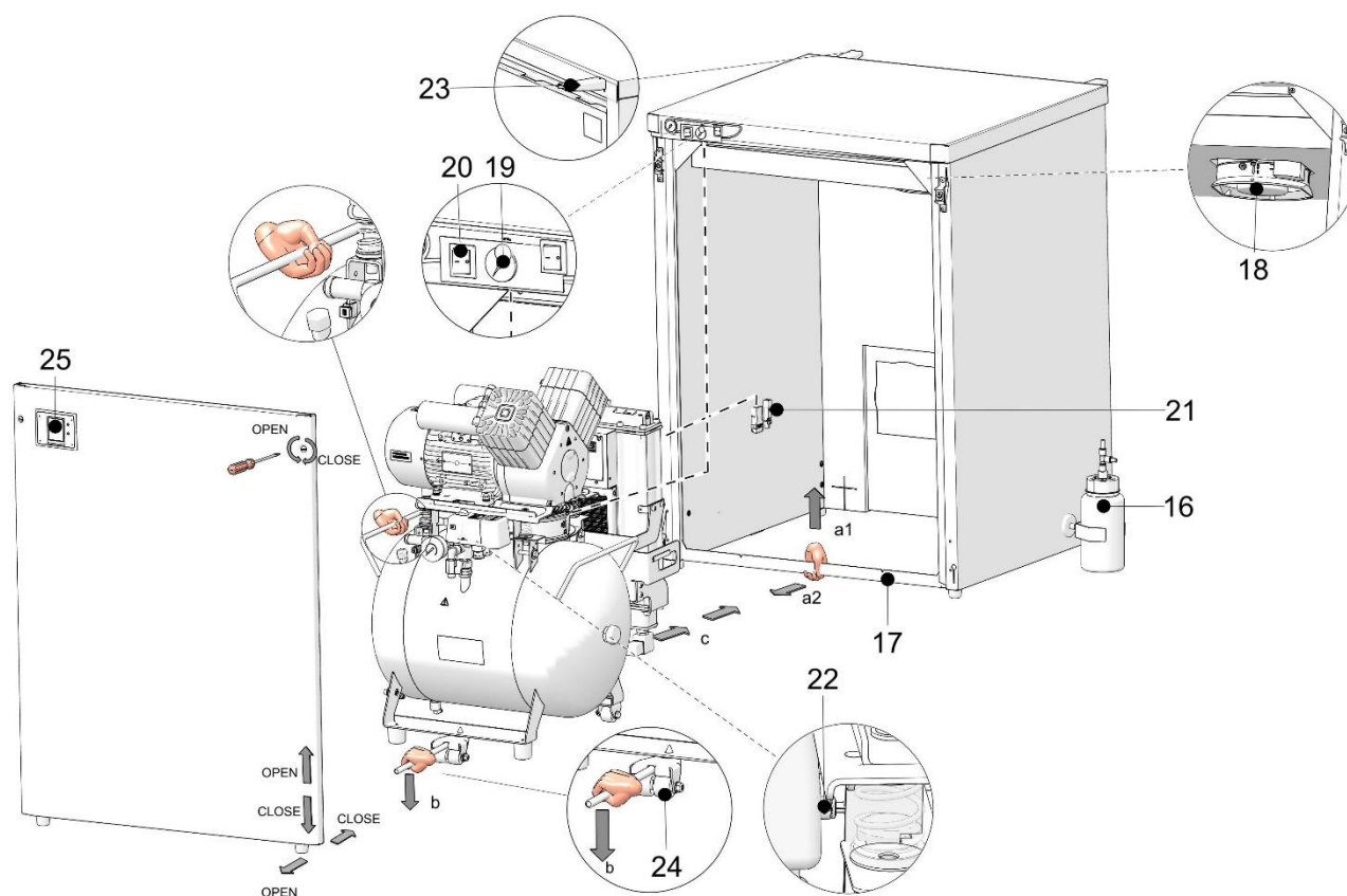
Obr. 4: Skrinka
