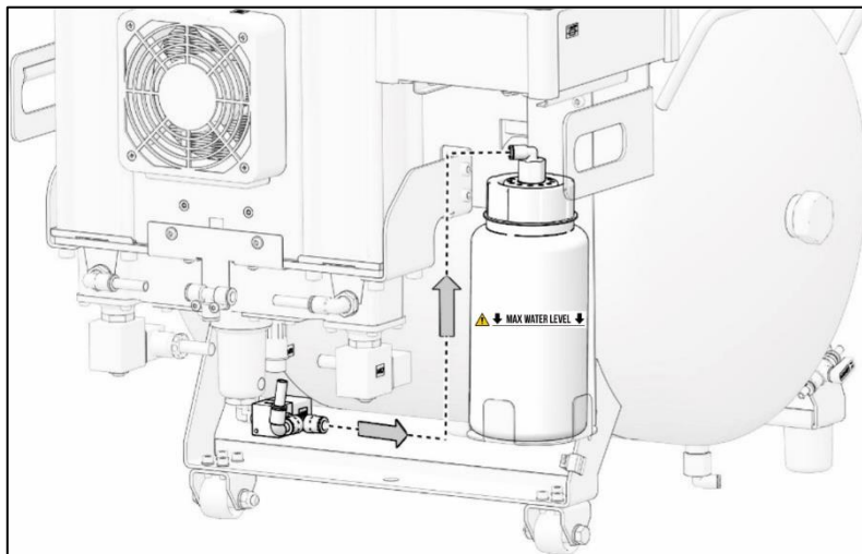
Abb. 23: Überprüfen des Kondensatauffangbehälters
